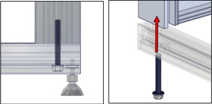
MFY-BOLT-375-16-2.5
